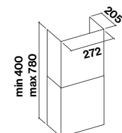
Optional chimney
