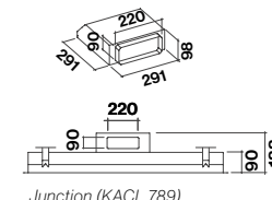
Junction (KACL.789)
