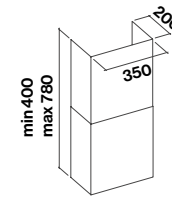
Optional chimney
