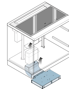
Under base h60 filter (KACL.951)
