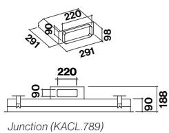
Junction (KACL.789)
