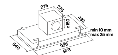
Junction (KACL.789)
